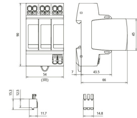
Maßbild DG MP YPV 1200 FM
