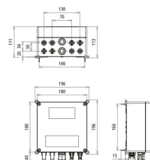
Maßbild DCU 2 YPV 1100 2M 1S MC4
