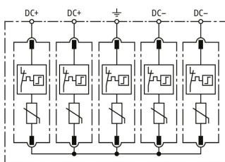
Prinzipialschaltbild DCU 2 YPV 1100 2M 1S MC4
