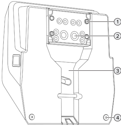
Abb. 4: Außenansicht (von hinten)
