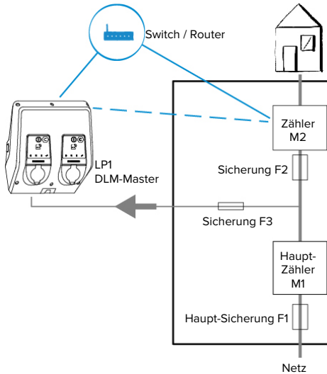
Abb. 26: Energiezähler misst nur externe Verbraucher
