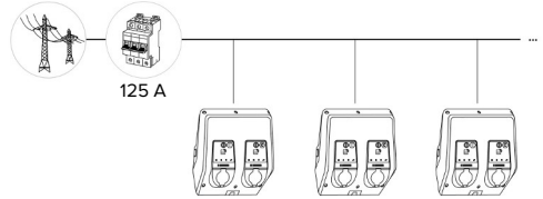
Abb. 19: Anschluss von mehreren Ladestationen über eine 125-A-Vorsicherung
