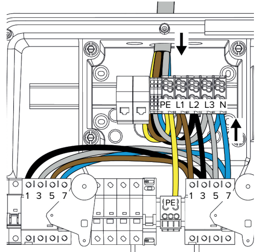
Abb. 18: Spannungsversorgung dreiphasig anschließen
