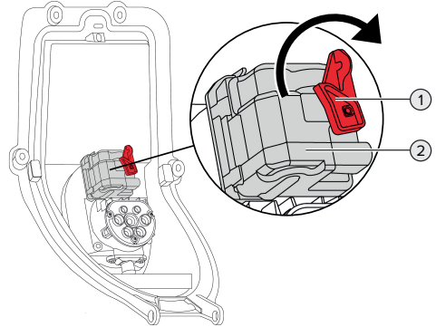
Abb. 35: Ladestecker manuell entriegeln
