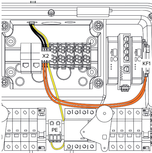
Abb. 21: Anschluss des Downgrade-Eingangs
