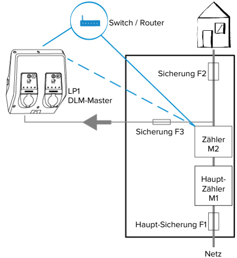
Abb. 27: Energiezähler misst externe Verbraucher und Ladestation (Gesamtverbrauch)
