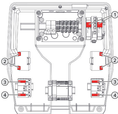
Abb. 7: Platzierung Eichsiegel (Produkt mit Ladesteckdose)
