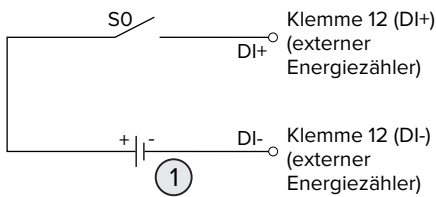
Abb. 28: Ansteuerung über ein Koppelrelais und einer zusätzlichen Spannungsversorgung
