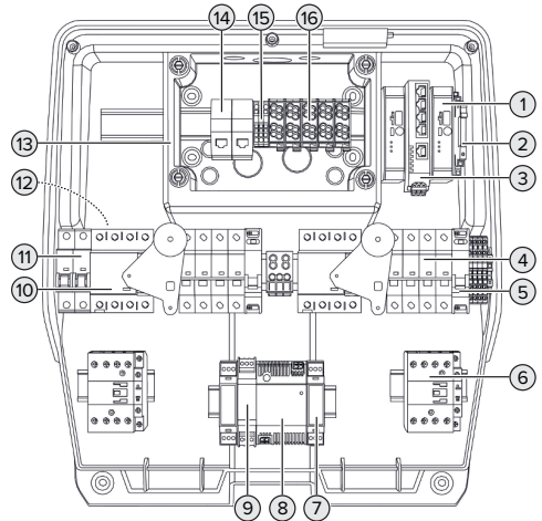
Abb. 5: Innenansicht
