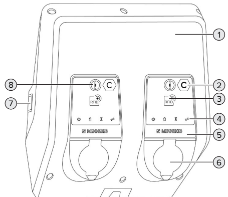
Abb. 3: Außenansicht (von vorne)
