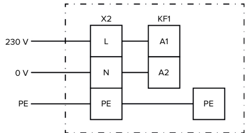
Abb. 20: Prinzipschaltbild: Anschluss eines externen Schaltkontakts
