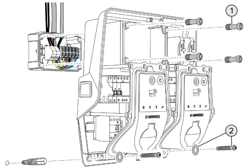
Abb. 17: Produkt montieren
