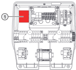
Abb. 23: Vorgesehener Bauraum für die Überspannungsschutzeinrichtung
