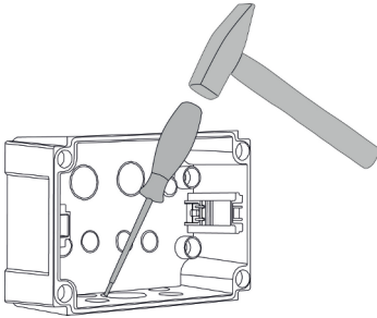
Abb. 14: Kabeleinführung herausschlagen (Beispiel)
