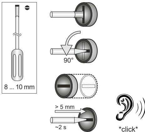
Abb. 33: Fehlerstromschutzschalter prüfen
