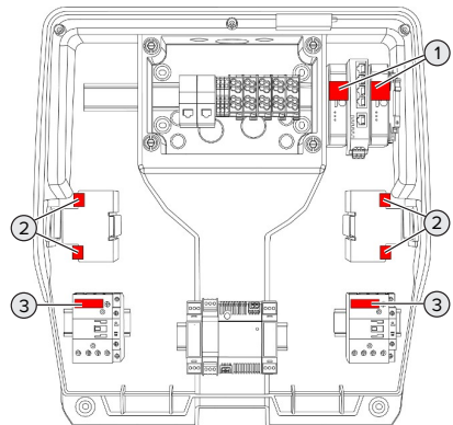
Abb. 8: Platzierung Eichsiegel (Produkt mit Ladekabel)
