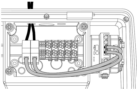
Abb. 22: Anschluss der Datenleitung (inkl. Durchschleifen)
