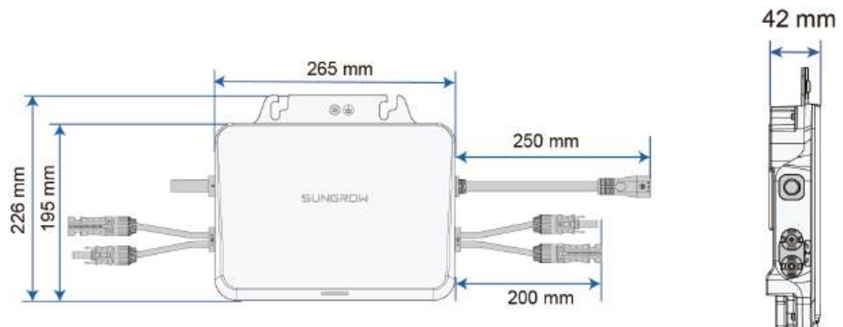
Abbildung 3-5 Abmessungen
