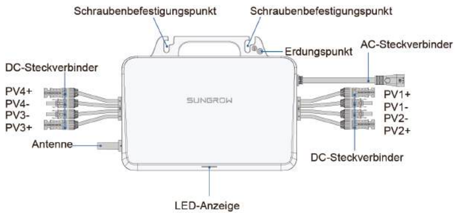
Abbildung 3-6 Äußerer Aufbau
