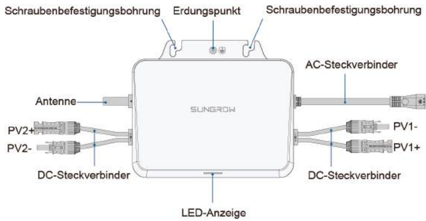
Abbildung 3-4 Äußerer Aufbau
