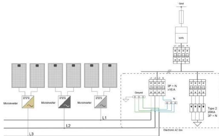
Abbildung 2-3 Systemschaltplan
