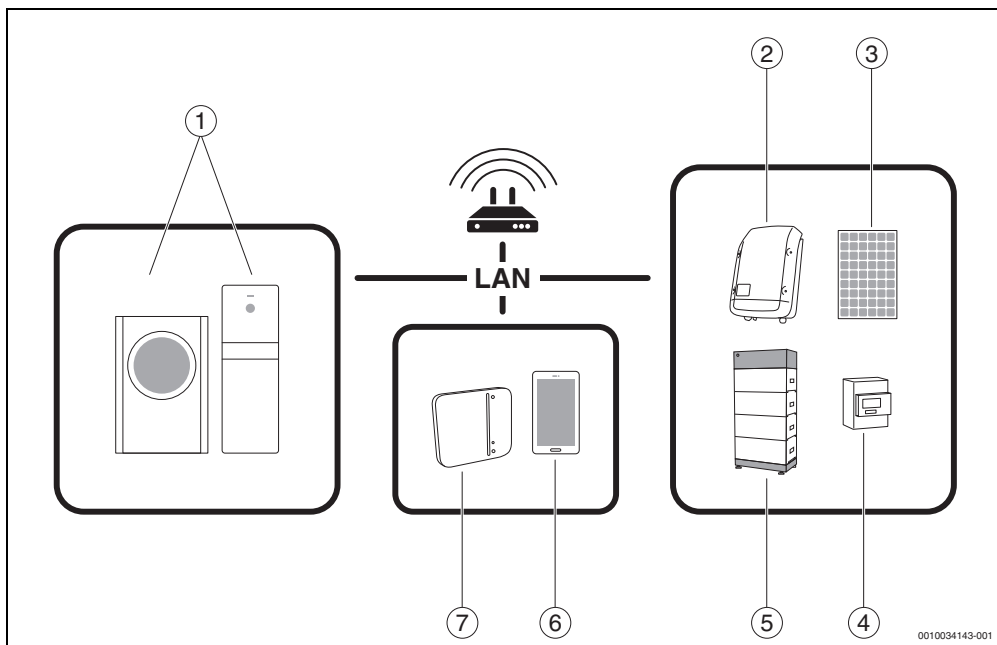
Bild 1 Systemübersicht
