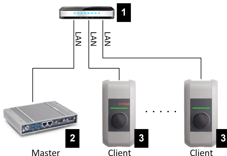
Abb. 2-5: Verbindung mittels Router oder Switch
