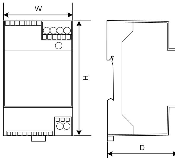
Abb. 11-20: Schematische Darstellung, Abmessungen in Millimeter
