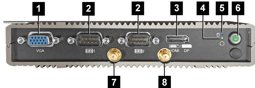
Abb. 3-6: Frontansicht Embedded PC
