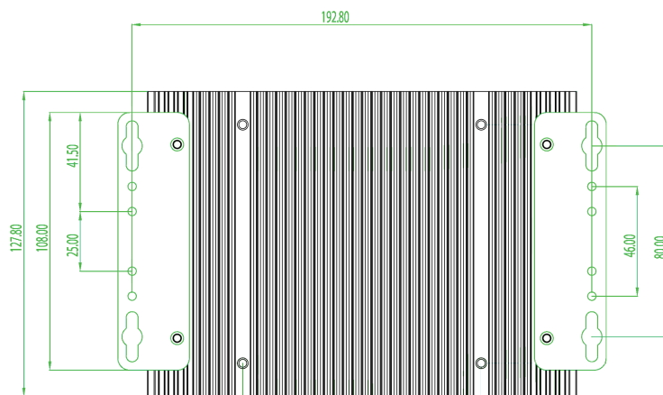
Abb. 5-10: Platzbedarf (in mm) bei Wandmontage
