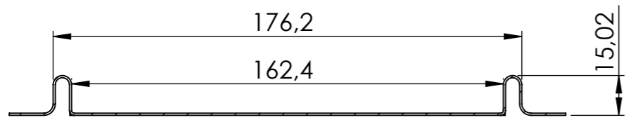
SCHNITT A-A MAßSTAB 1 : 2
