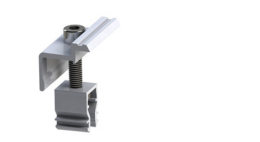
Endklemme Click ohne Pin Produktnummer: 802304C
