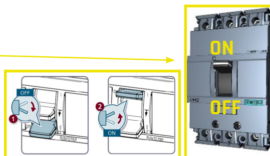
Abb. 25: Lasttrennschalter
