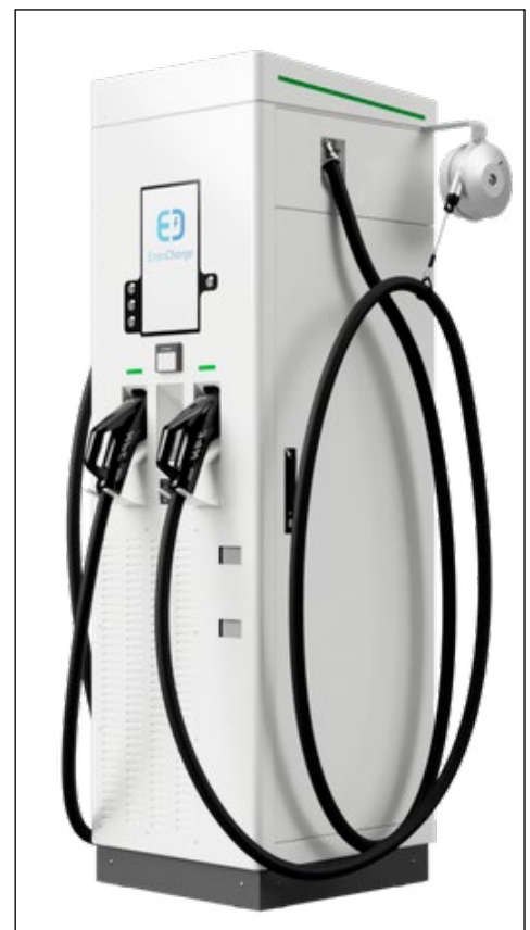
Abb. 45: ECC 320 Vorderansicht
