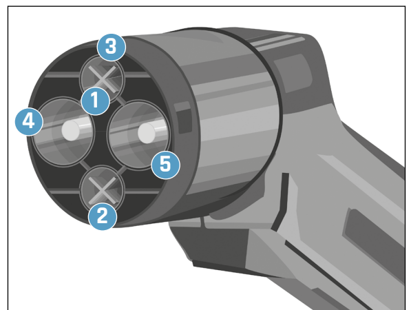
Abb. 48: CHAdeMO Ladestecker
