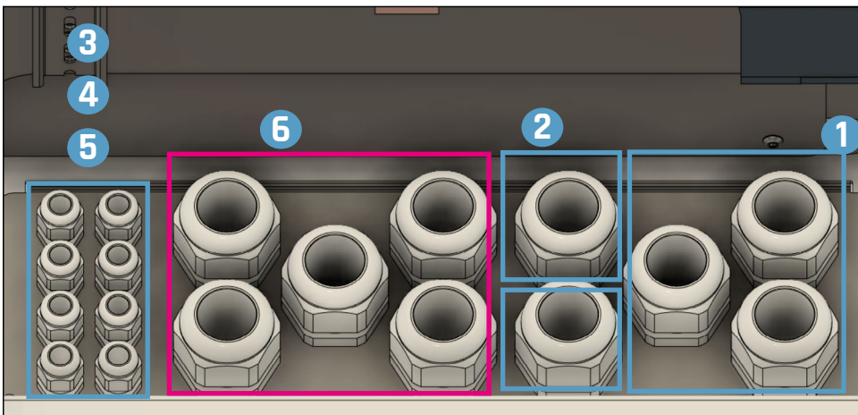
Abb. 28: Kabelbelegung Kabeldurchführungsplatte
